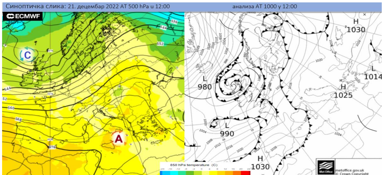
Синоптичка ситуација за 21. децембар 2022.
