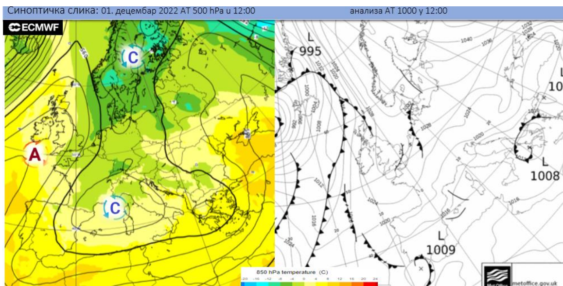
Синоптичка ситуација за 1. децембар 2022.
