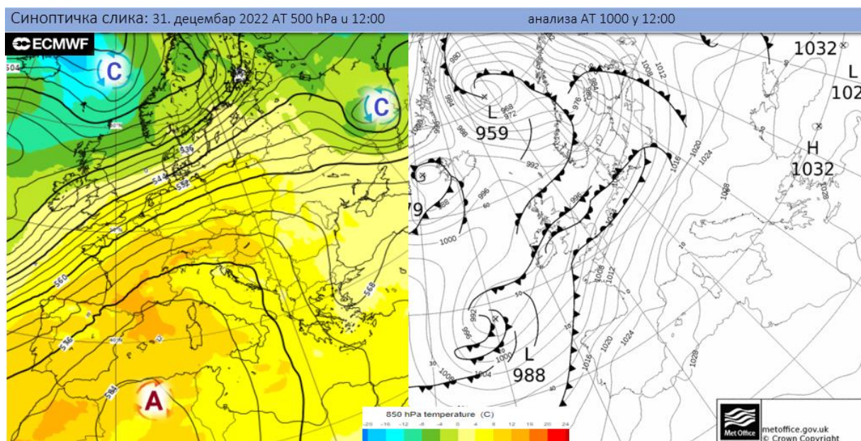
Синоптичка ситуација за 31. децембар 2022.
