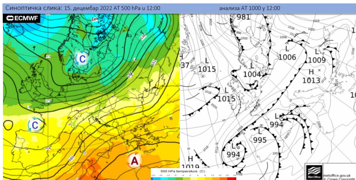
Синоптичка ситуација 15. децембар 2022.
