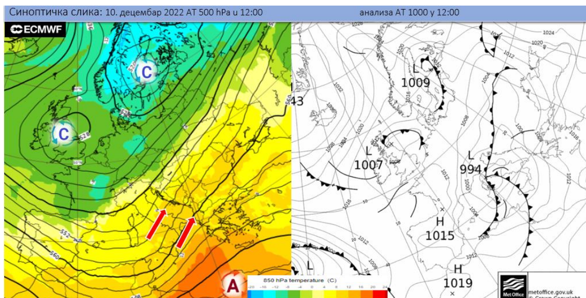
Синоптичка ситуација за 10. децембар 2022. године
