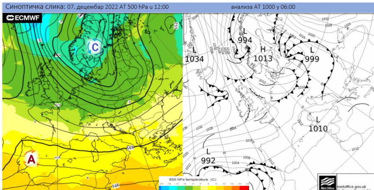
Синоптичка ситуација за 7. децембар 2022. године
