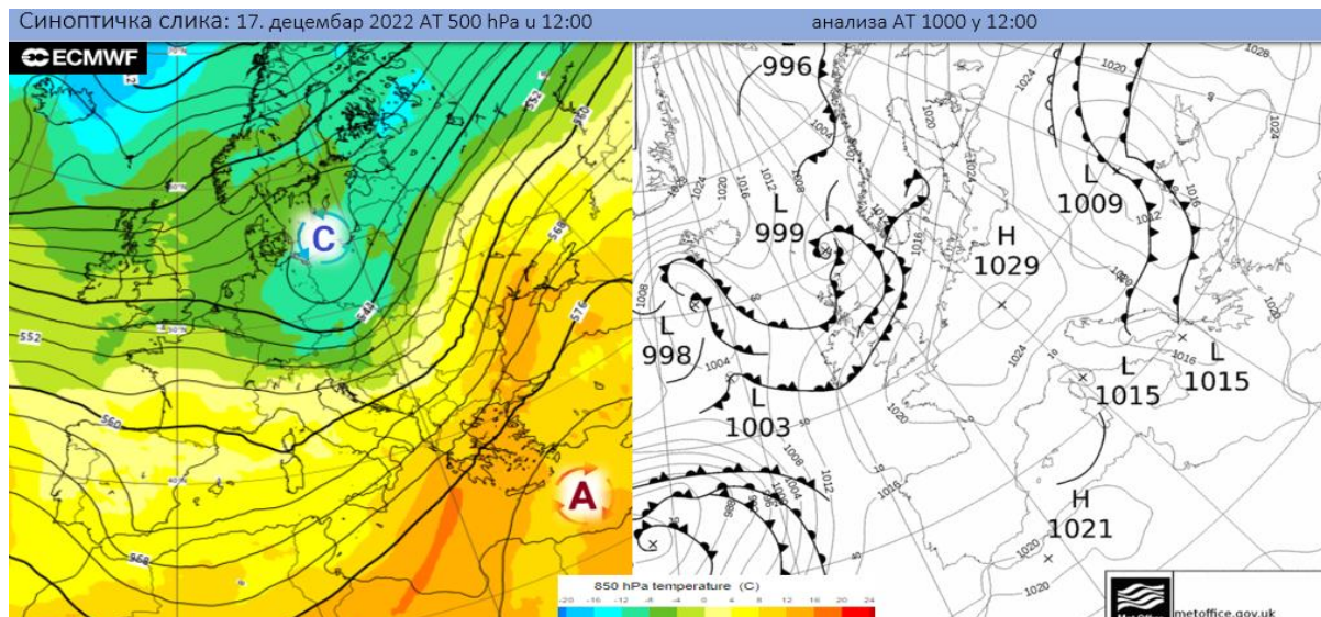
Синоптичка ситуација за 17. децембар 2022.
