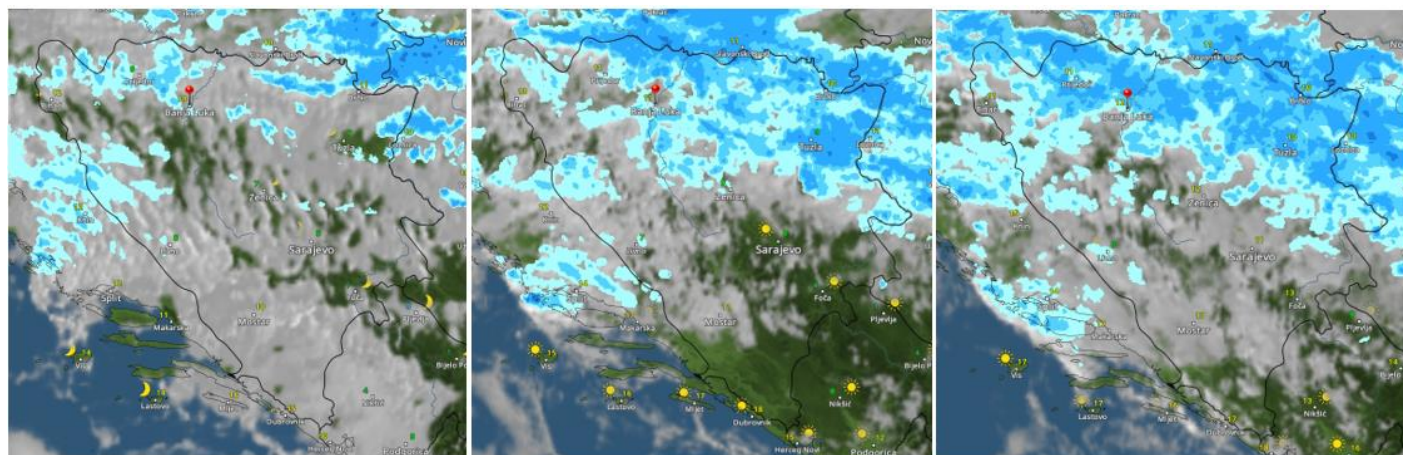
Синоптичка ситуација за 27. децембар 2022.
