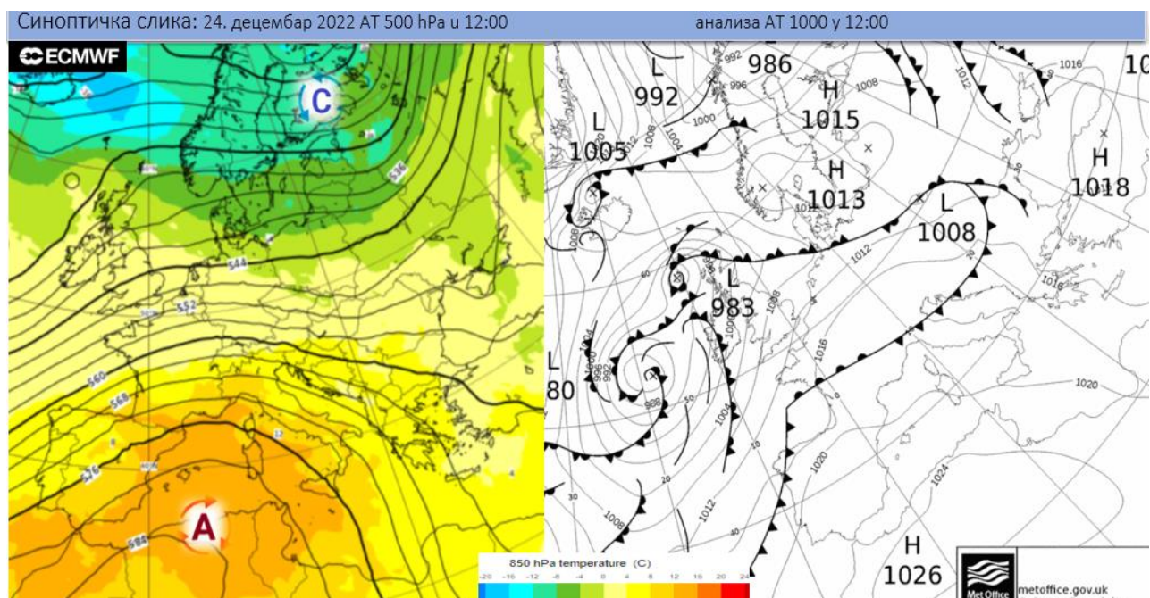
Синоптичка ситуација за 24. децембар 2022. године
