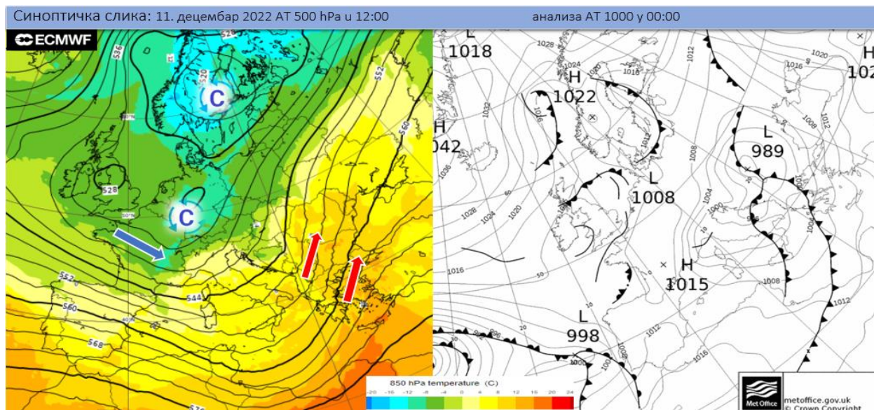
Синоптичка ситуација за 11. децембар 2022. године
