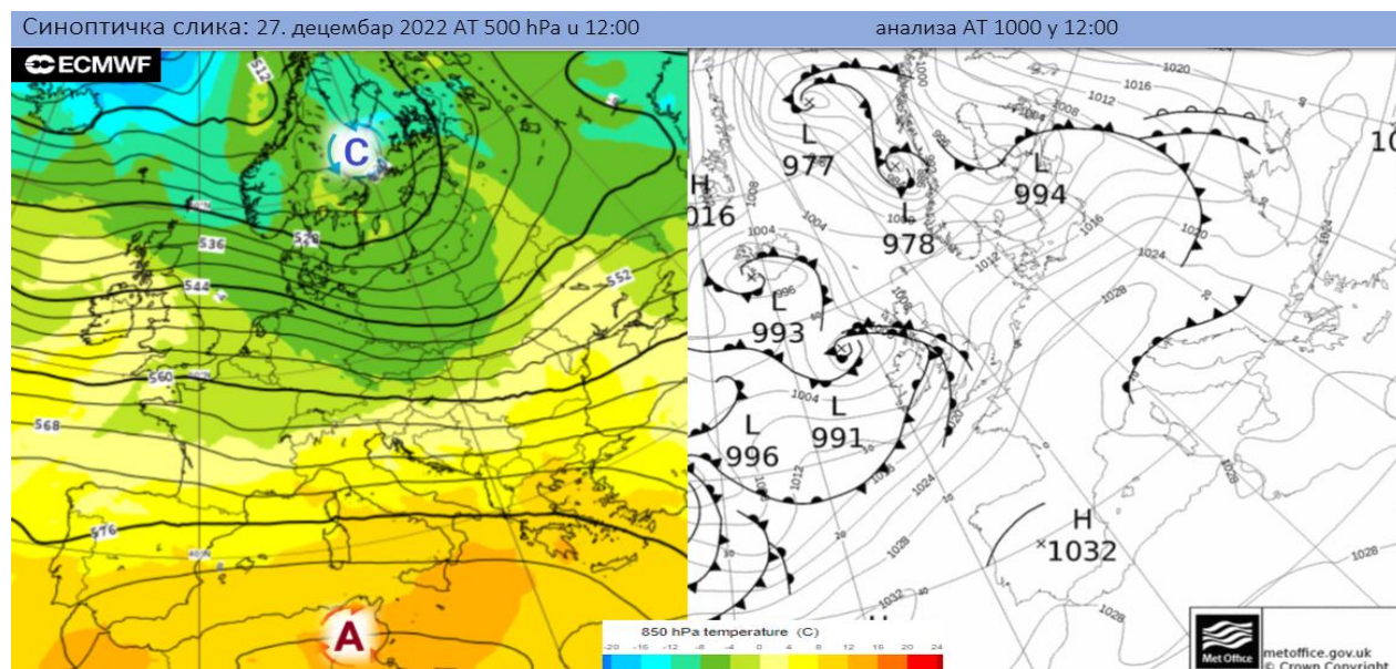
Синоптичка ситуација за 27. децембар 2022.
