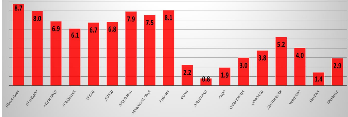
Одступање средње максималне температуре у односу на просјек у 3.декади децембра 2022.
